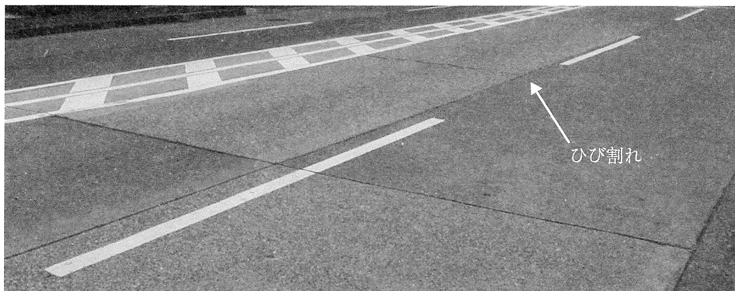
写真 4-1 ひび割れの状況
