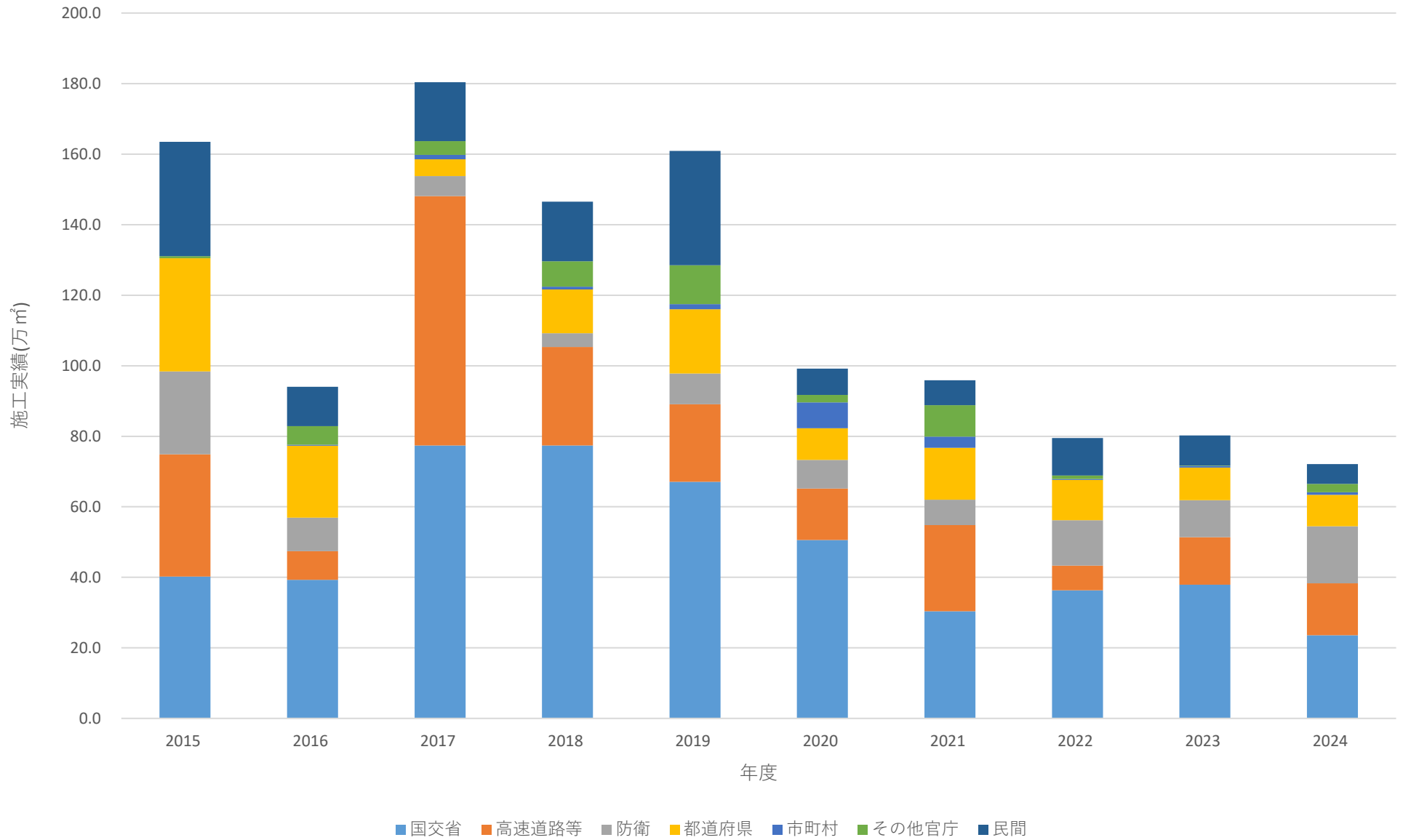
コンクリート舗装の施工実績(発注機関別)
