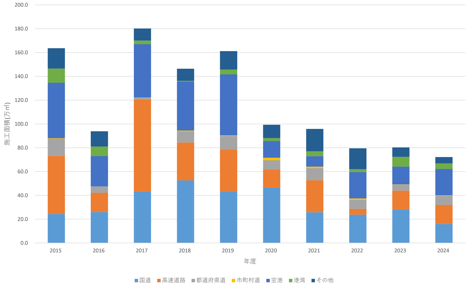
コンクリート舗装の施工実績(適用場所別)
