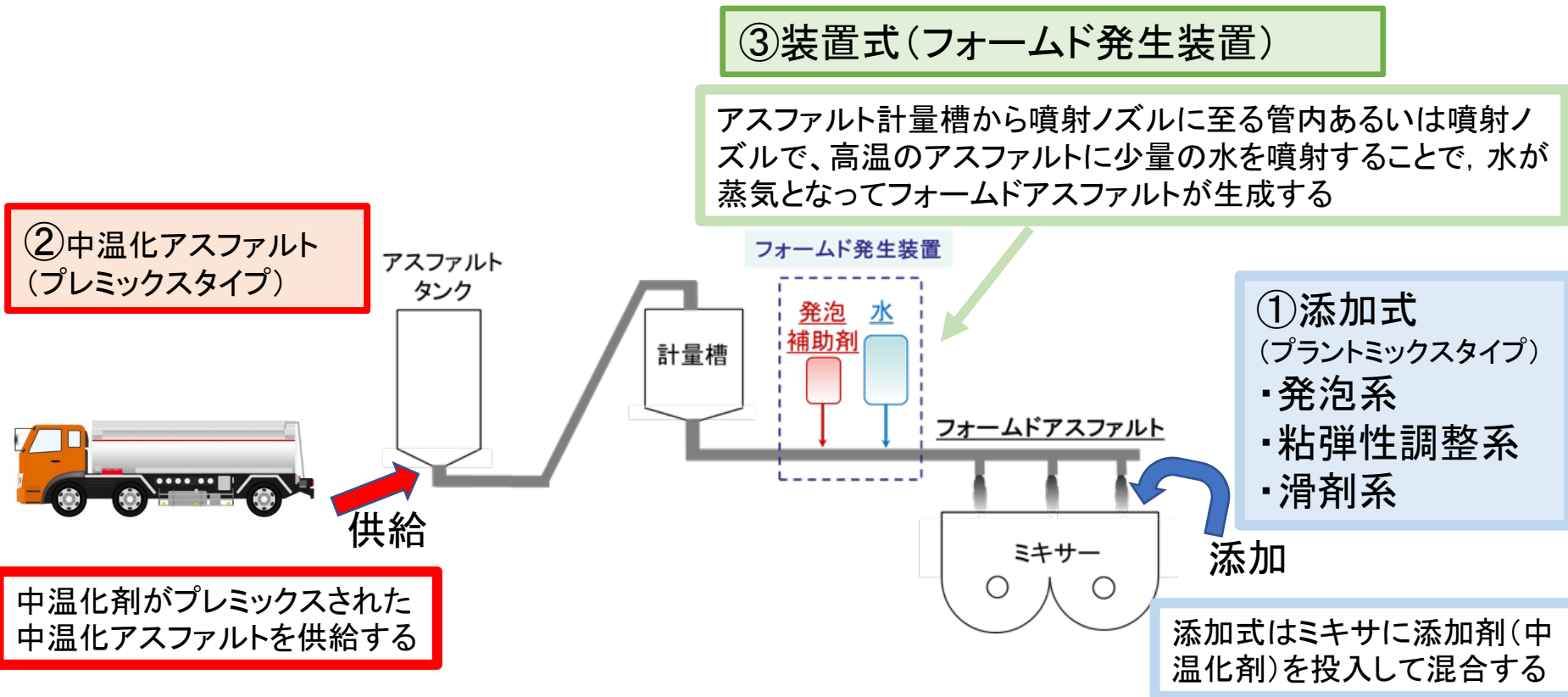
図- 中温化技術の概要
