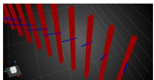
3Dモデルによる 既設アンカーと 計画H鋼の干渉 チェック
